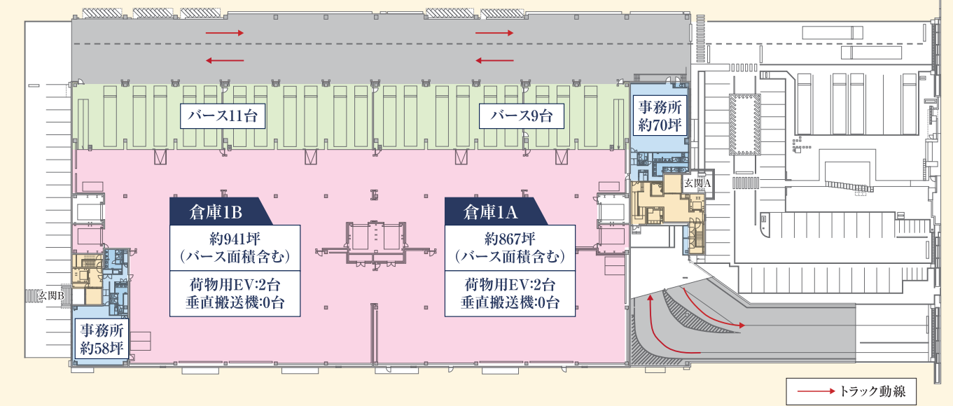
2階 平面図 双方向通行も容易な車路幅の確保
