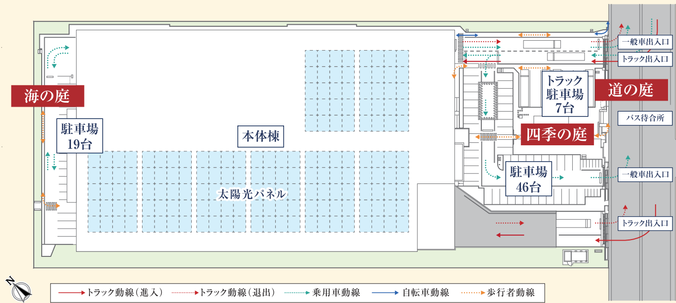
配置図 1階2階バスへの独立動線 大型待機場7台完備
