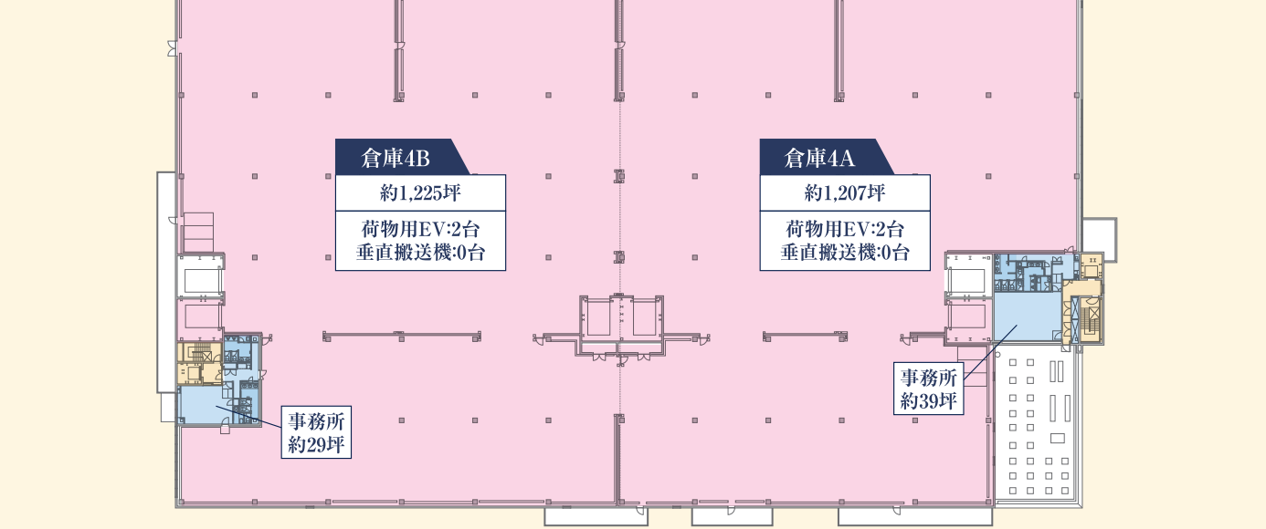
4階 平面図 最大8基の上下搬送機が迅速なオペレーション支援
